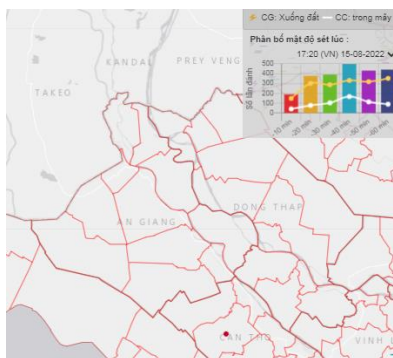
Ảnh vệ tinh định vị sét
