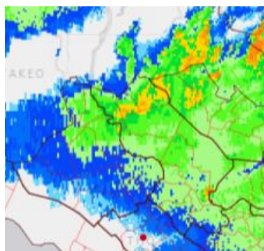
Ảnh Radar phản hồi mây
